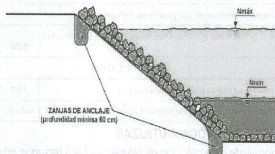
Figura: Protección tipo escollera
