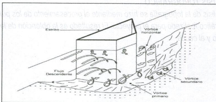
Figura: Socavación local de un estribo
