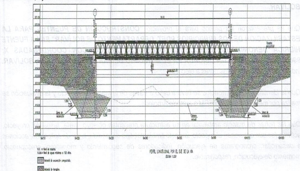
Figura: Perfil de la obra a ejecutar
