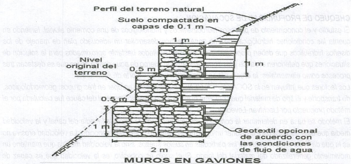
Figura: Esquema típico de muros de gaviones protección cauce.
