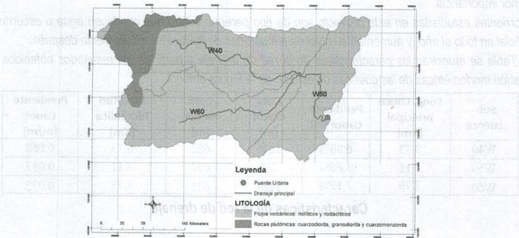
Figura. Formaciones geológicas de la zona de estudio
